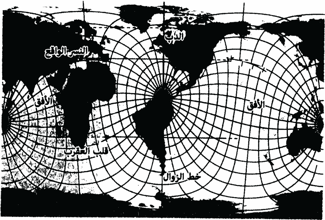
الشكل (66): مسارات قلب العقرب والنسر الواقع والذئب للفترة نفسها كما في الشكل (62) بالنسبة إلى مراقب في كاراكاس في فنزويلا.
